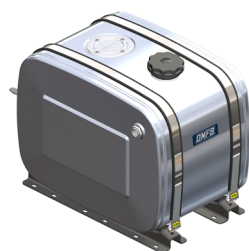
Serbatoio retro-cabina completo di kit Rear cab tank + kit assembly
