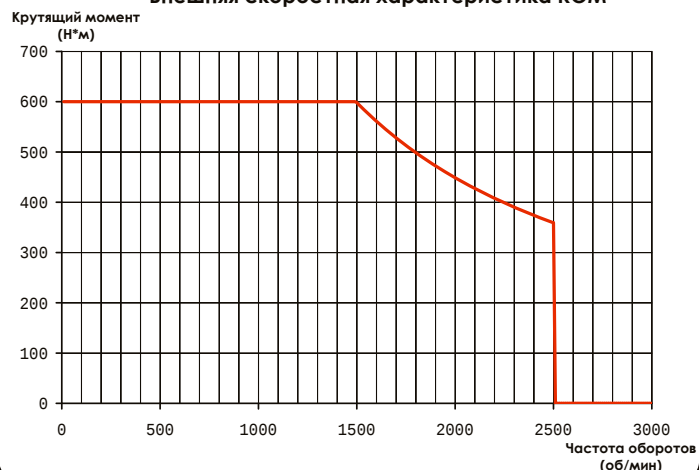
Внешняя скоростная характеристика КОМ
